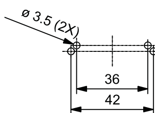
USINAGEM P/ EIXAÇÃO DO MANCAL
