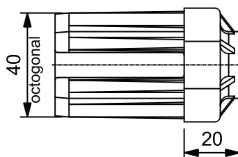
PONTEIRA C/ FURO
