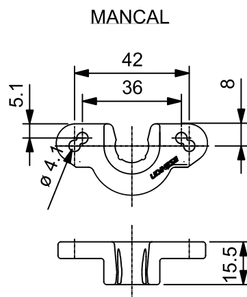
USINAGEM P/ EIXAÇÃO DO MANCAL
