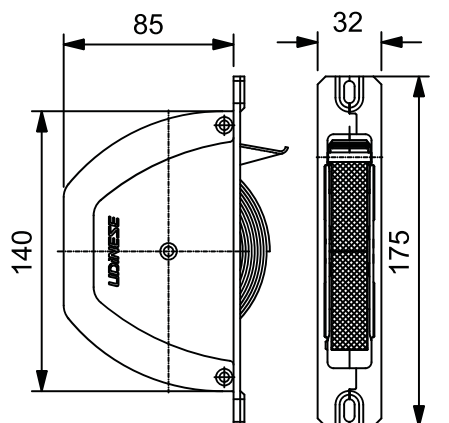
CAIXA DO RECOLHEDOR
